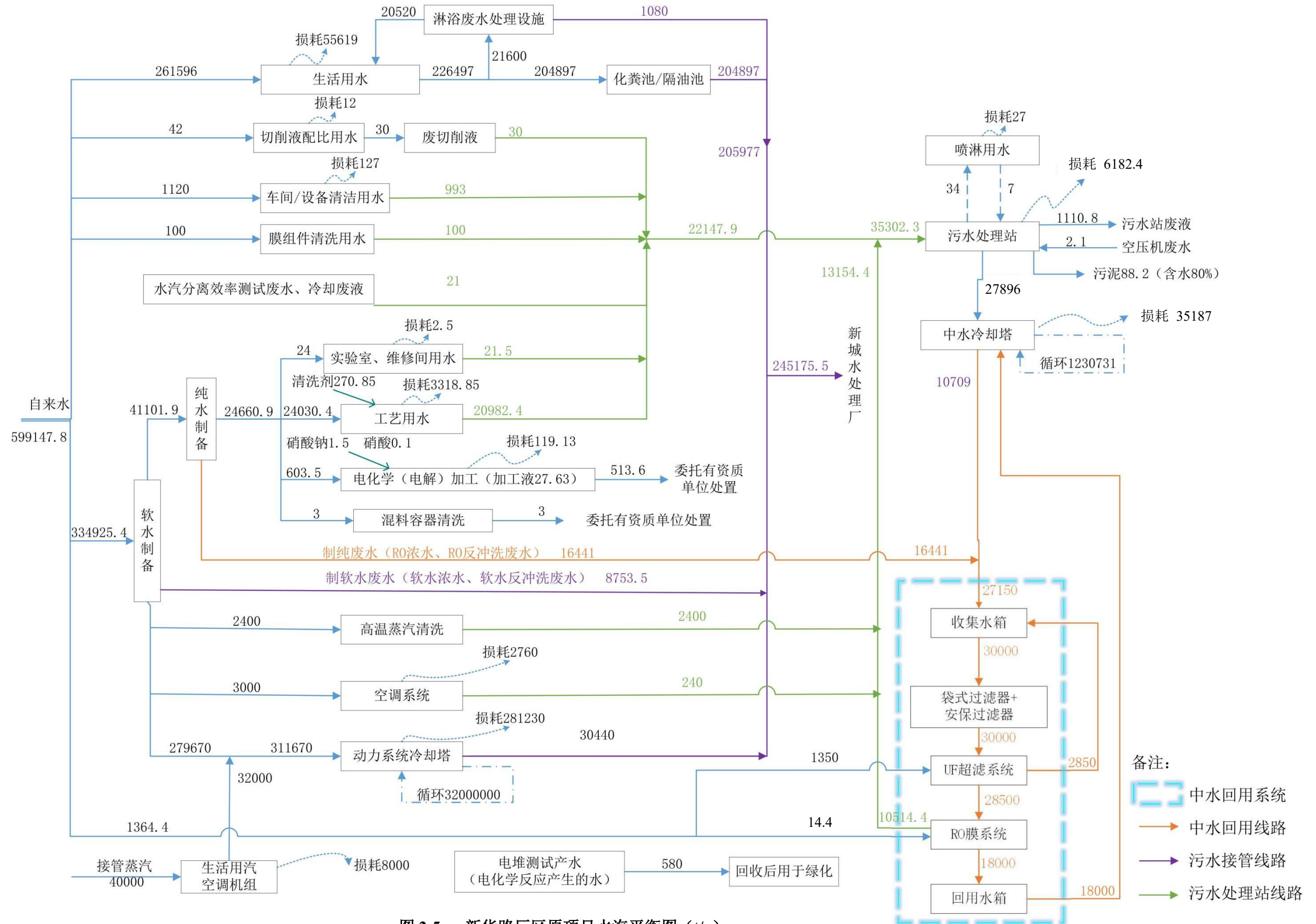
图 2-5 新华路厂区原项目水汽平衡图 (t/a)
